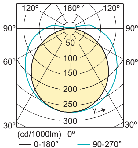
LEDtube PERF 10.5 W /865 600 mm T8 I
