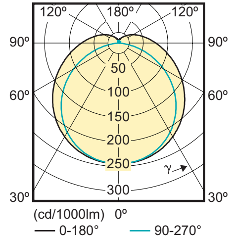
LEDtube VLE 600 mm 10 W T8 ROT
